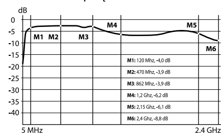
Tłumienność sprzężenia WE→SAT
